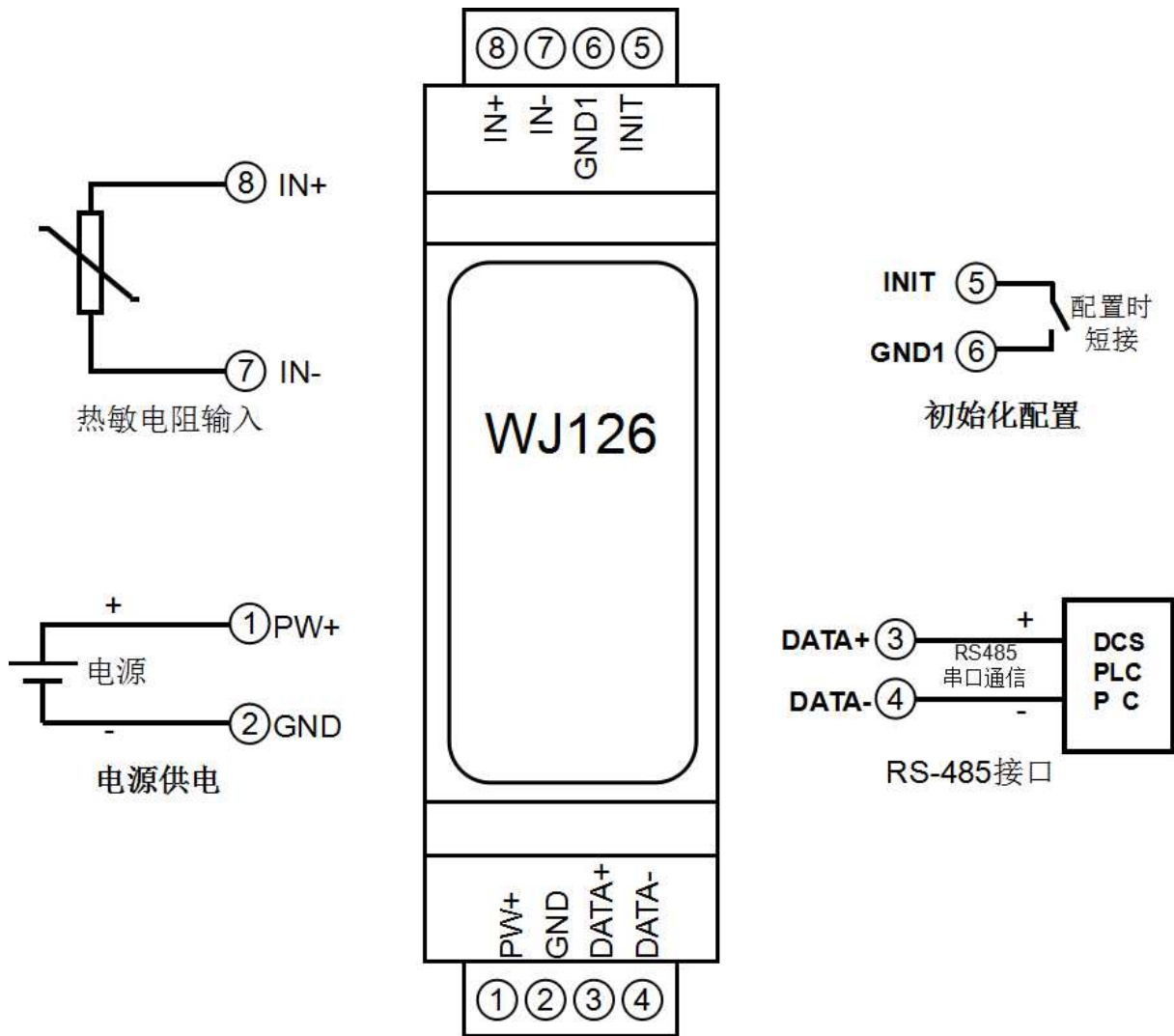
图3 WJ126 模块接线图
