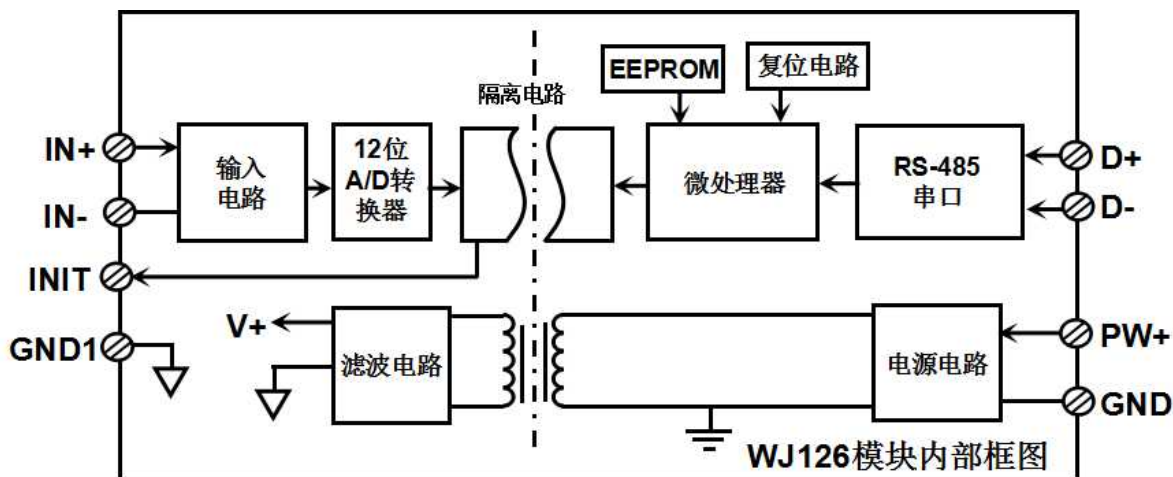
图2 WJ126 模块内部框图
